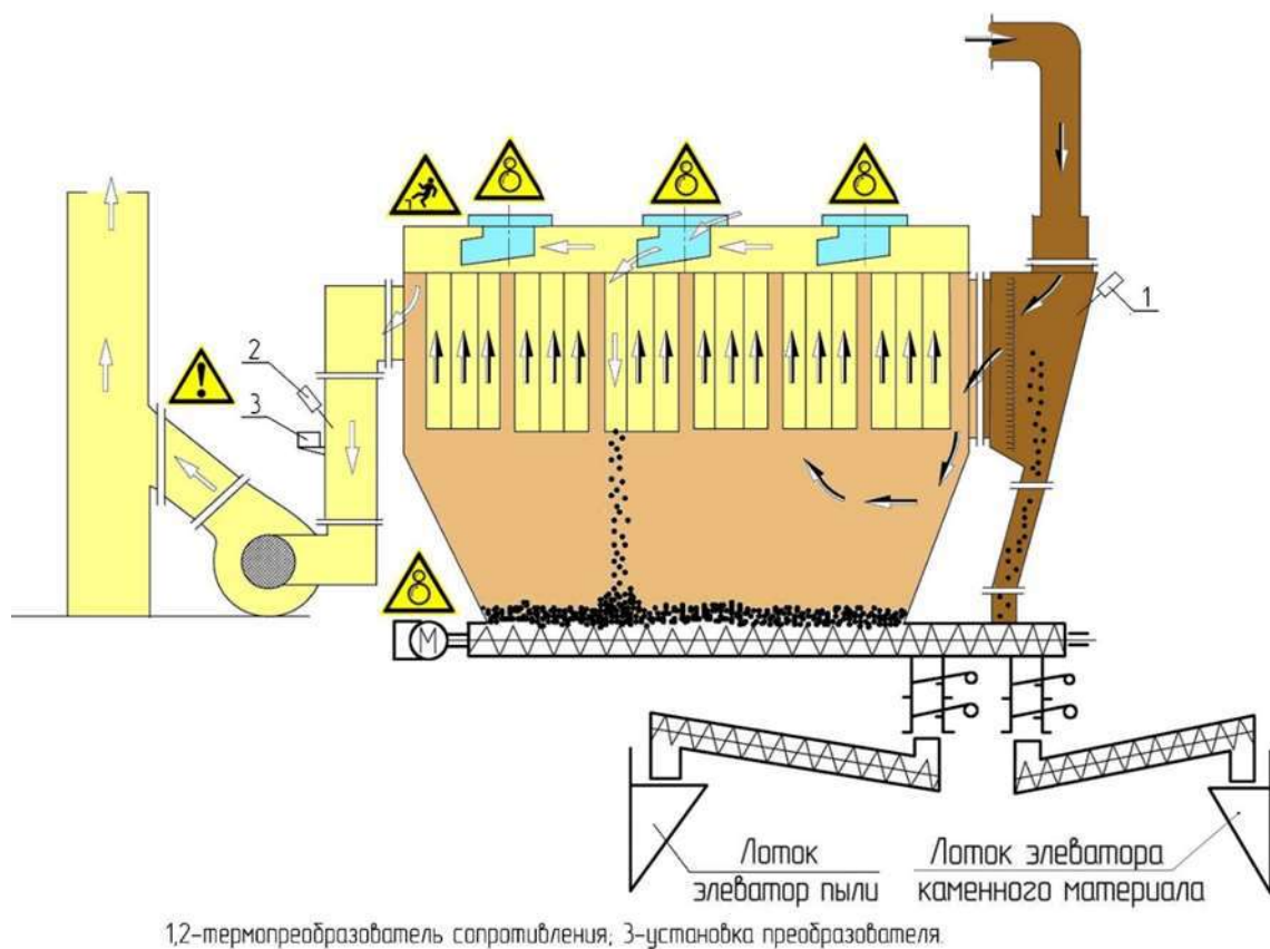
Схема технологическая установки рукавного фильтра
