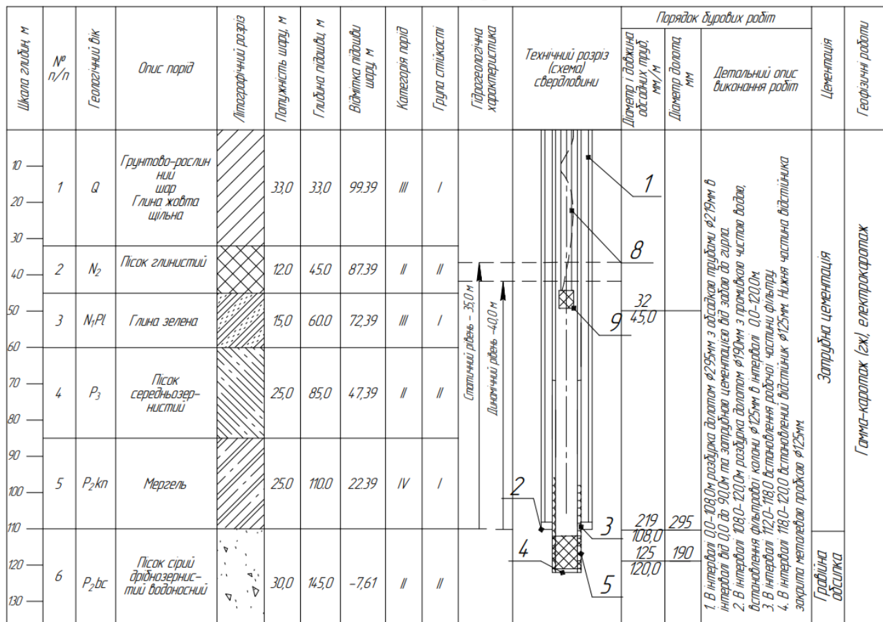
Рис. 1.4 – Геологічний розріз і конструкція свердловини
