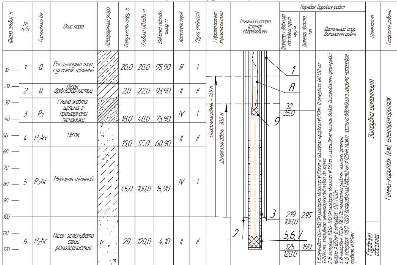
Рис. 1.5 – Геологічний розріз і конструкція свердловини
