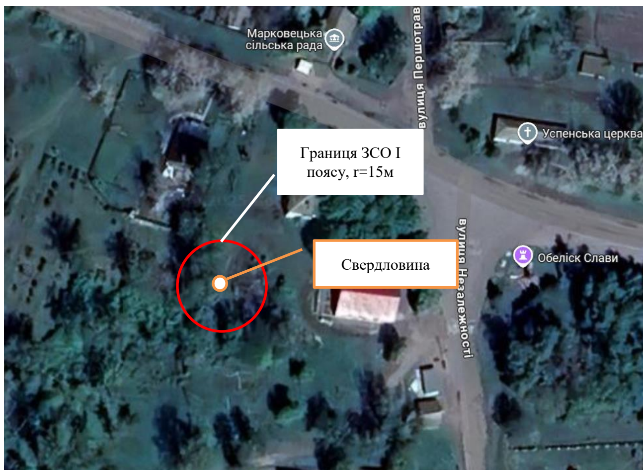
Рис. 7.1 Ситуаційний план розміщення ЗСО I поясу
